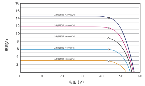
曲线特性图 (SYMN156R02TBD-680W)
