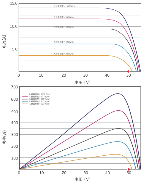
曲线特性图 (SYM156TBDO-650W)
